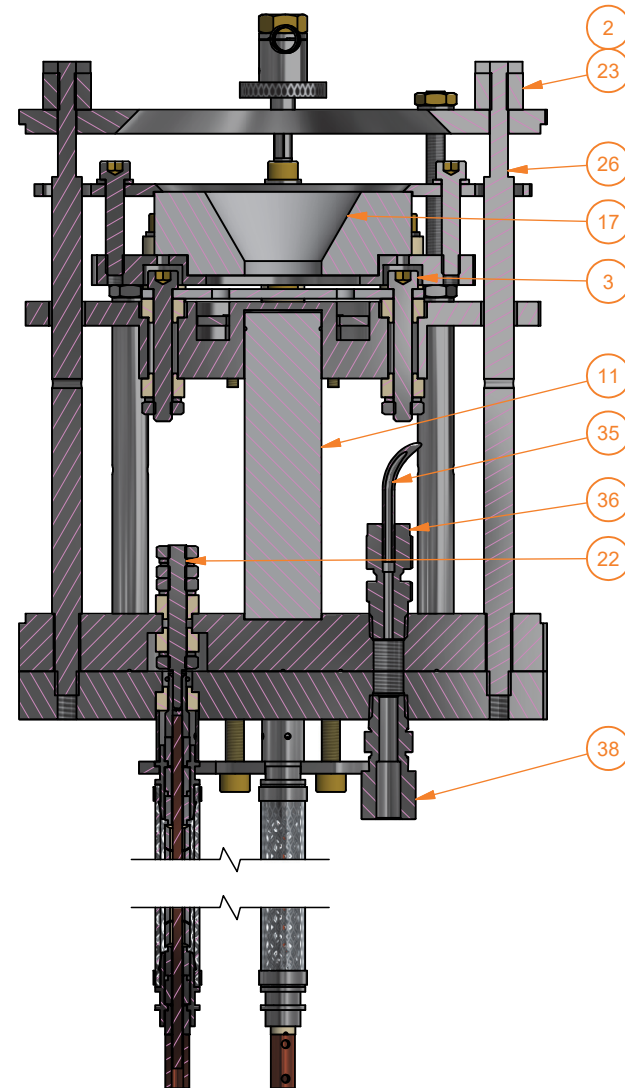
SECTION D-D SCALE 1:2
